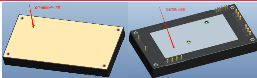
模块铝基板热点温度位置示意图
