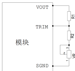
图 9 Trim 调压接线图
