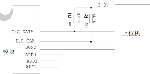
图 6 上位机连接图
